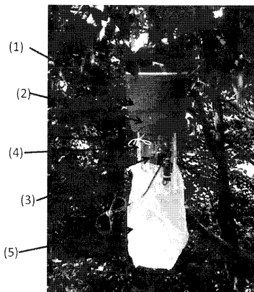
Figura 1: trappola tipo CDC modificata a CO 2 .
