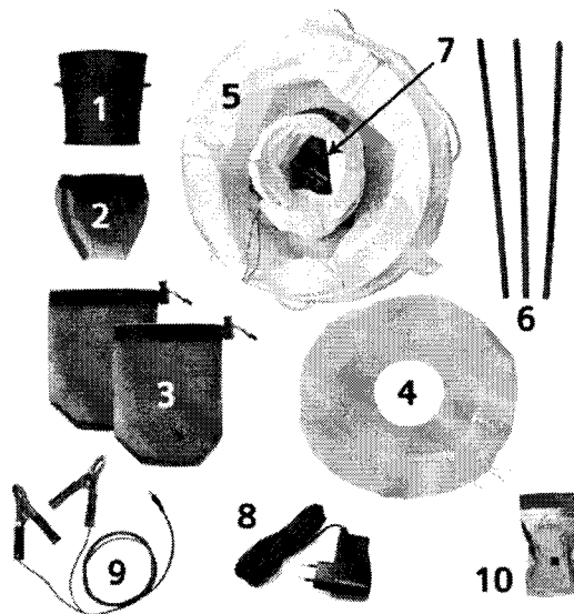
Figura 6: trappola BG-Sentinel non assemblata.
